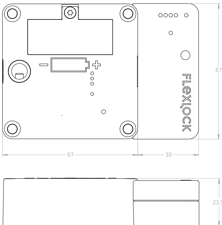
FLEXLOCK INVISIBLE MED CARD+ BLUETOOTH-MODUL
